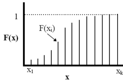
Figura 4. Função de distribuição acumulada.
